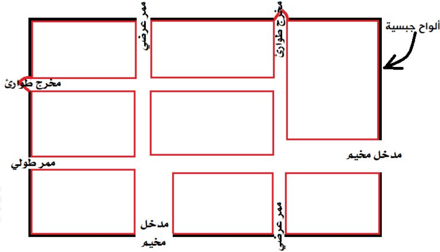
طريقة تركيب الألواح الجبسية على السياج الخارجي للمخيمات
